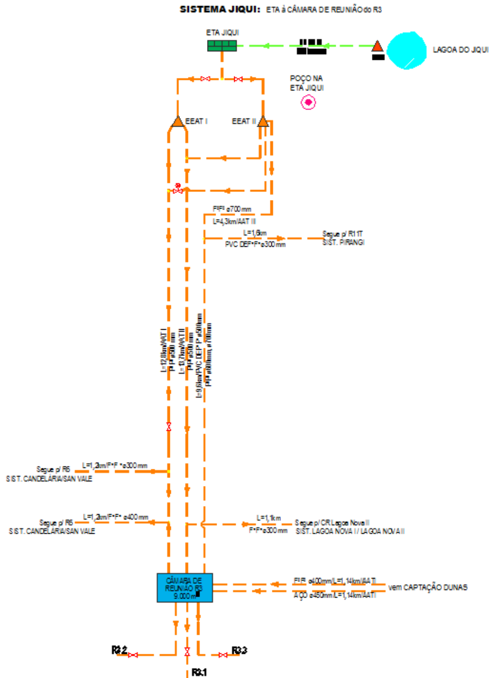
Figura 11. Sistema Jiqui: ETA à Câmara de Reunião do R3
