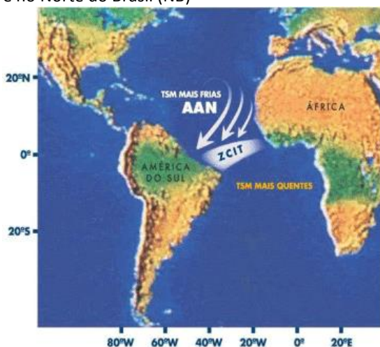
Figura 61. TSM no oceano Atlântico e influência da ZCIT com anos chuvosos a muito chuvosos no NEB e no Norte do Brasil (NB)
