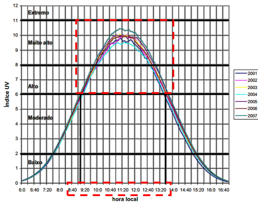
Figura 74. Gráfico do índice de UV com médias horárias anuais em função da hora local de junho de 2001 a dezembro de 2007, com destaque aos horários em que há máxima atuação aos níveis alto e muito alto da escala de eritema.
