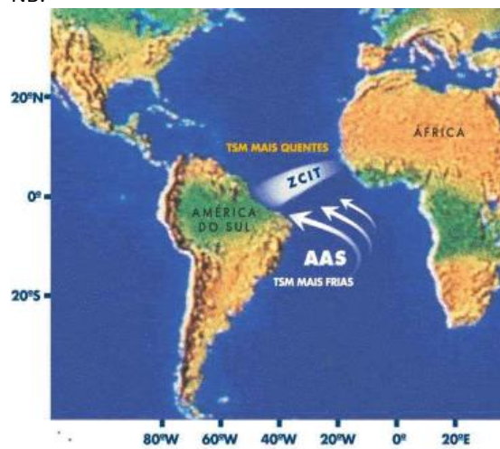
Figura 62. TSM no oceano Atlântico e influência da ZCIT com anos secos ou muito secos no NEB e no NB.
